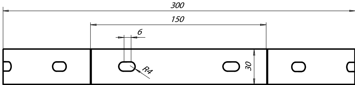
Seitenansicht
