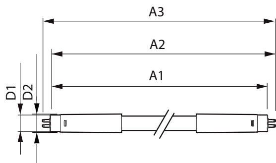
MAS LEDtube HF 600mm HO 8W865 T8
