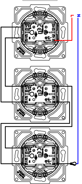
Bağlantı Şeması / Wiring Diagram
