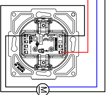
Bağlantı Şeması / Wiring Diagram
